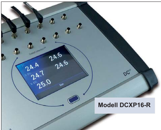
DCXP16-R mit speziellen Eingangsbuchsen kompatibel mit den Driesen+Kern "rugged Datenloggern" aus der, rugged plus , DK3XX- und DK6xx- Serie
